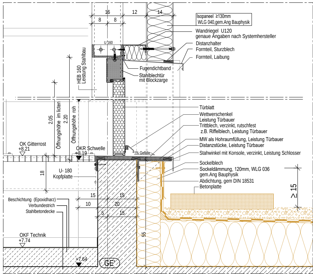
DETAIL 1 M. 1:10
