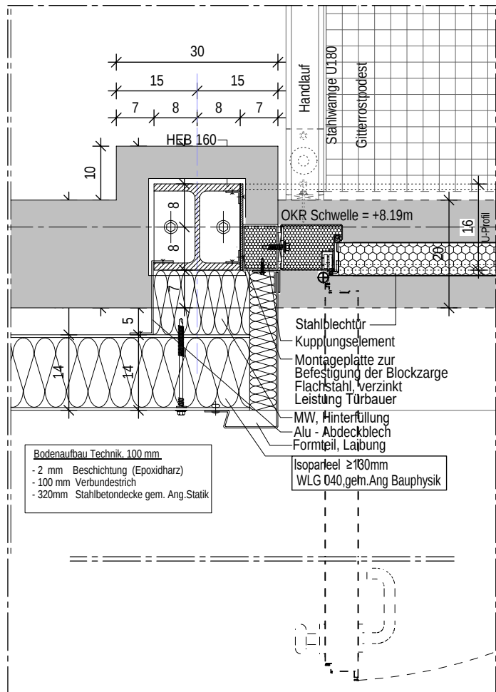
DETAIL 2 M. 1:10
