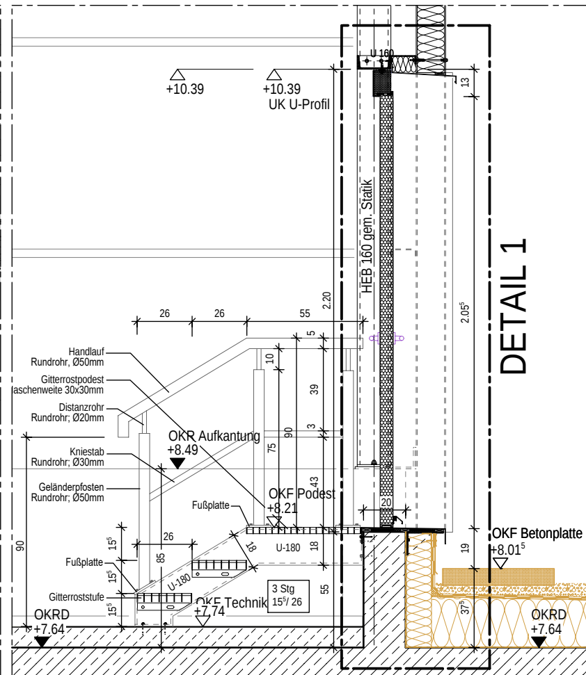
SCHNITT M. 1:25
