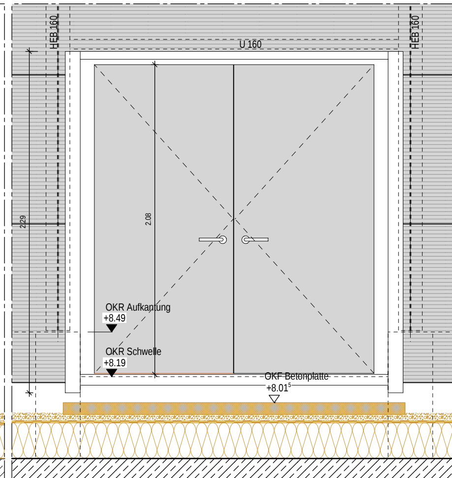
ANSICHT M. 1:25
