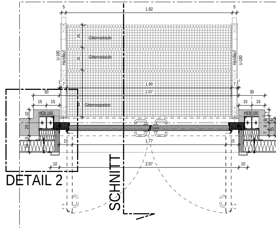
GRUNDRIS M. 1:25
